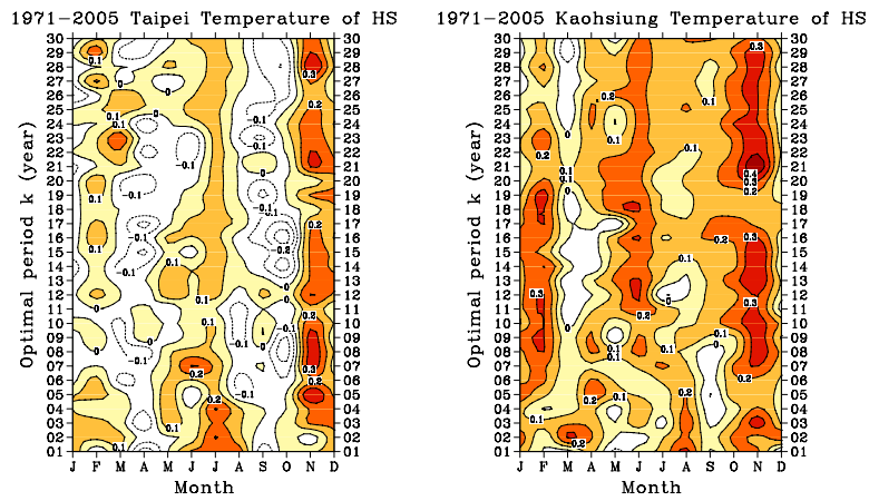
圖1. 台北、高雄測站在1971-2005年預報期之不同K年與不同月份HSS技術得分之分佈圖，x軸代表月份，y軸代表K年。
