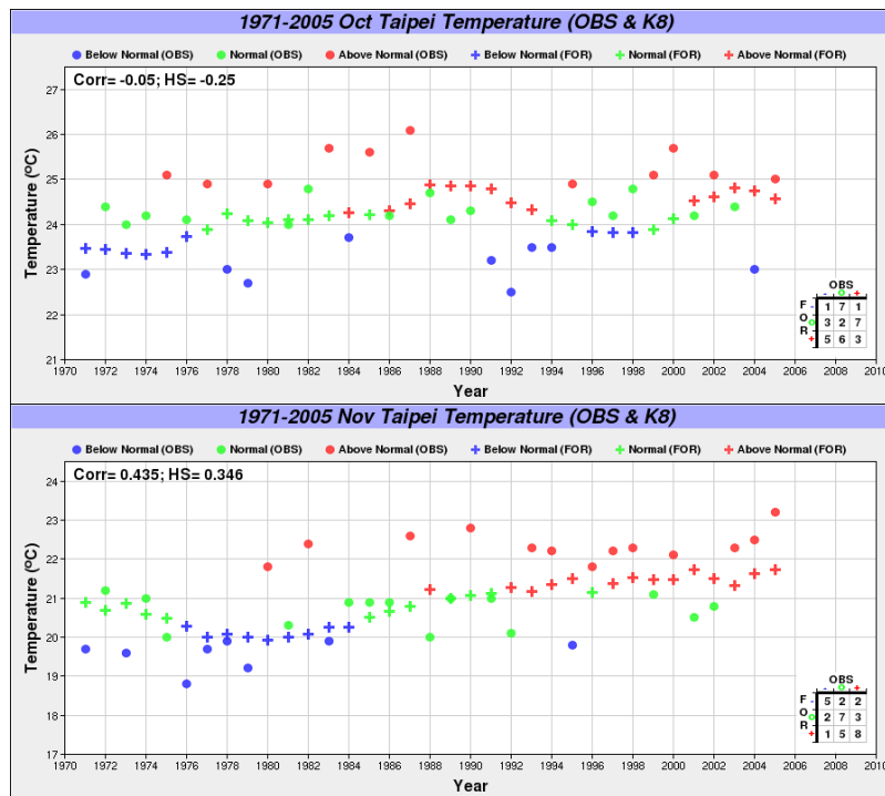
圖2. 1971-2005年台北測站溫度10月、11月之觀測與預報之時間序列圖。圖中●代表觀測值，+代表預報值，藍色為Below Normal，綠色為Near Normal，紅色則為Above Normal，右下角則是HSS的三分類技術得分表。
