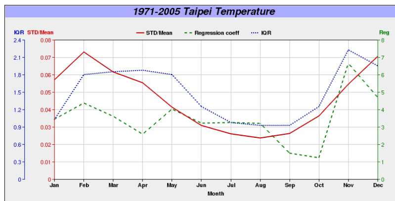
圖3. 台北測站觀測溫度之標準差/平均值、迴歸係數值、IQR的1-12月時間序列圖。圖中IQR代表所有資料(1971-2005年)的百分之75的值減去百分之25的值。
