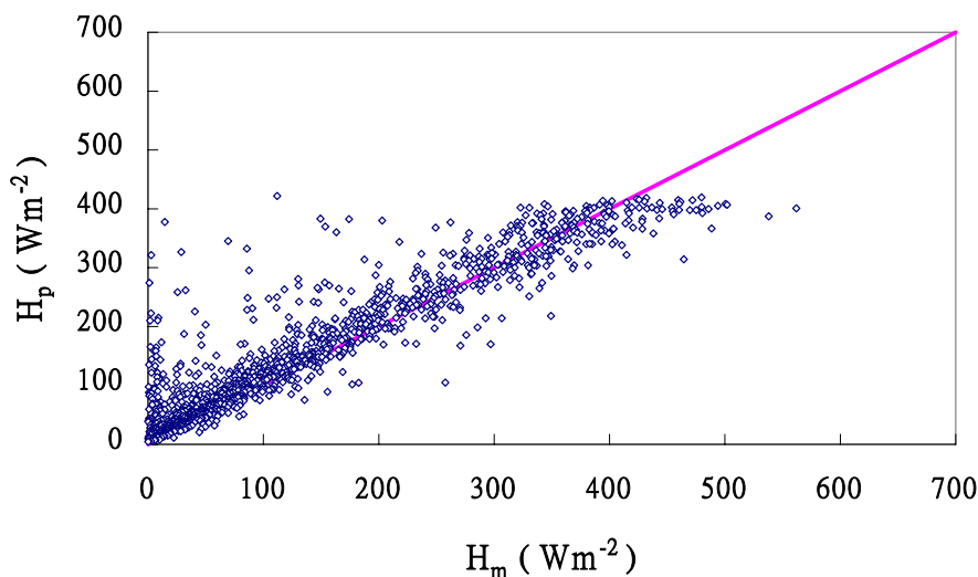
圖一、可感熱通量比較圖，以森林為例：通量變化法預測值( H_p )與渦流相關法測得之可感熱通量( H_m )比較圖。
