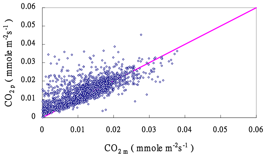
圖二、二氧化碳通量比較圖，以森林為例：通量變化法預測值( \text{CO}_{2\text{ p}} )與渦流相關法測得之二氧化碳通量( \text{CO}_{2\text{ m}} )比較圖。
